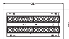
295*145 AW-GSD 10-2
